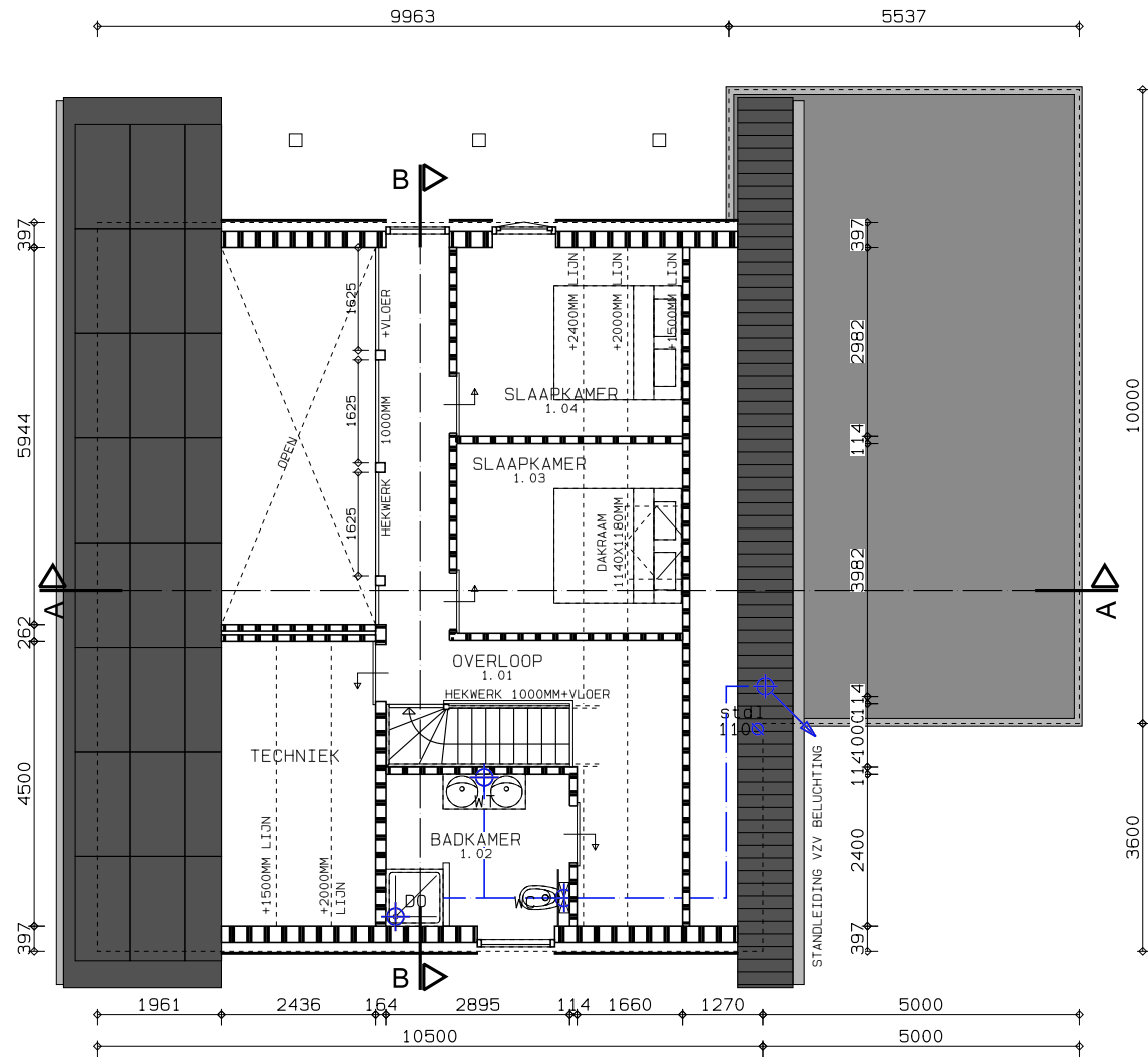
VERDIEPING
